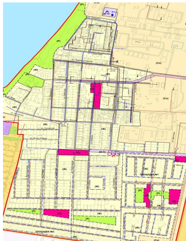
Рисунок 2.4.9.2 - Размещение перспективных объектов системы водоснабжения на территории посёлка, ПЛОЩАДКИ №1 и №3
